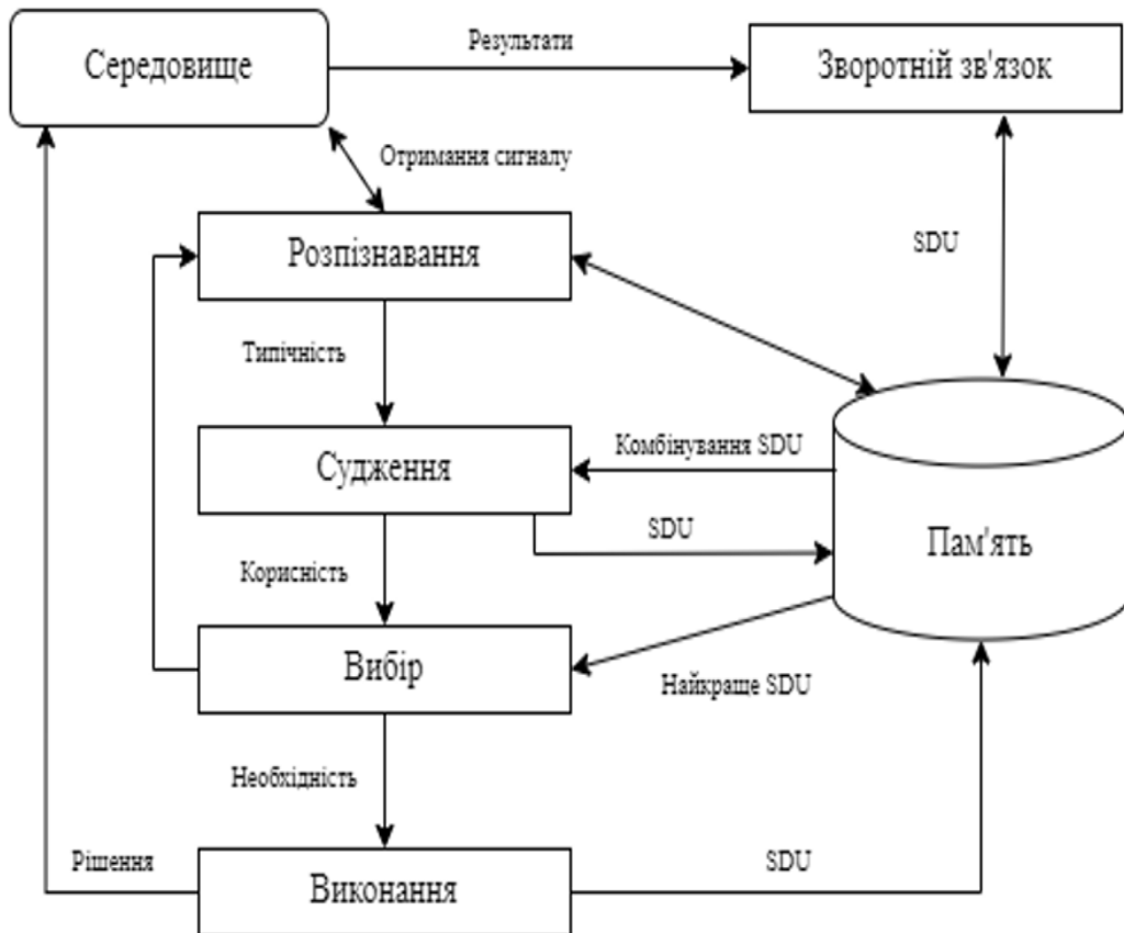
Рис. 2. Архітектура IBLT
