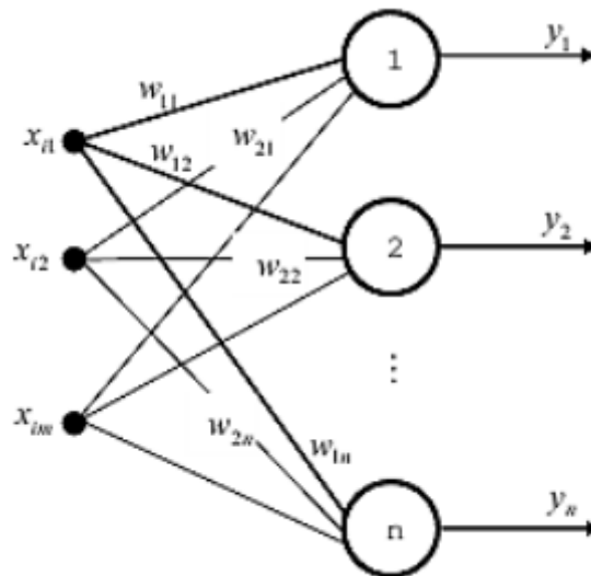
Рис. 4. Структура мережі Кохонена
