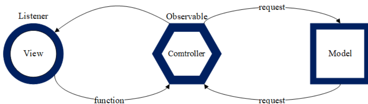
Рис. 4. Графічне представлення роботи GetX
