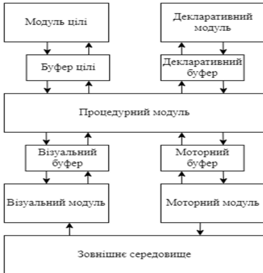
Рис. 1. Архітектура АСТ-R
