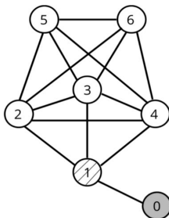
Рис. 5. «Граф-квітка», у якого 7 вершин та 14 ребер
